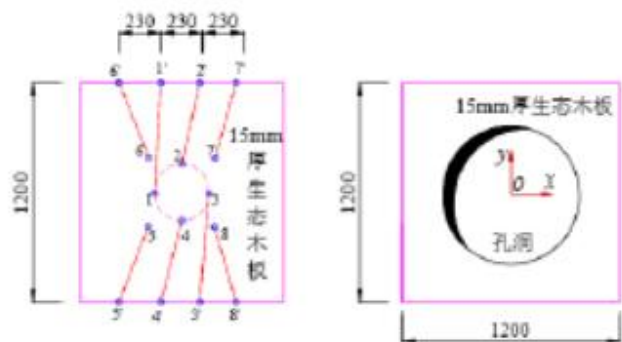
附图3 加载台平面图
